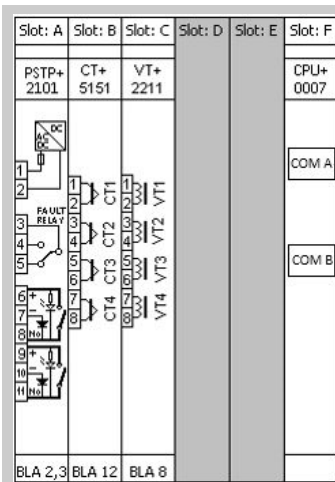
Equipement S24/Fr & S24/L
