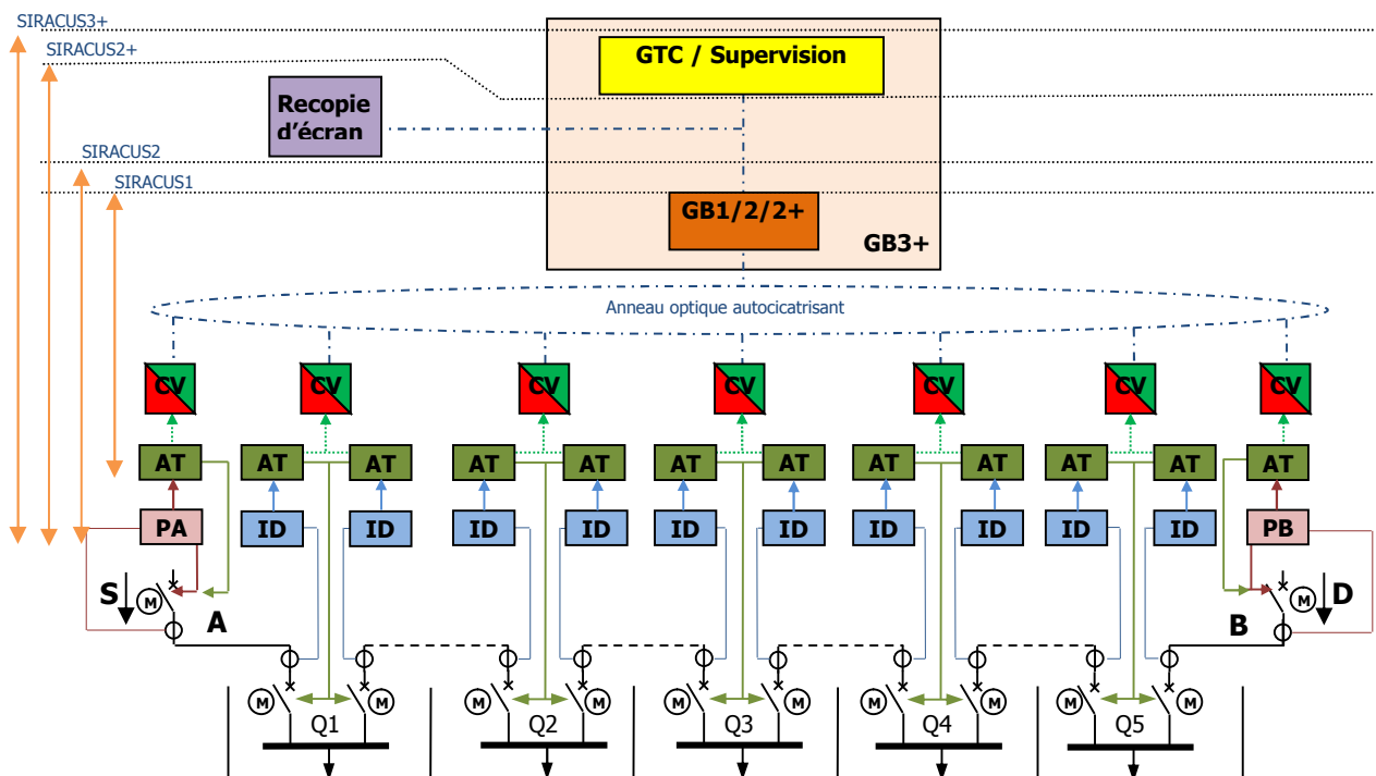
Systèmes de Reconfiguration Automatique de Boucle SIRACUS1 - SIRACUS2 - SIRACUS2+ - SIRACUS3
