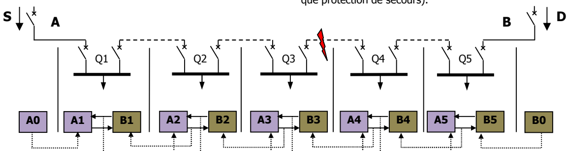
Schéma de principe de SIRACUS MANU Chaque relais voyant le défaut bloque ses deux voisins. Le relais ne recevant qu'un ordre de blocage déclenche le disjoncteur.
